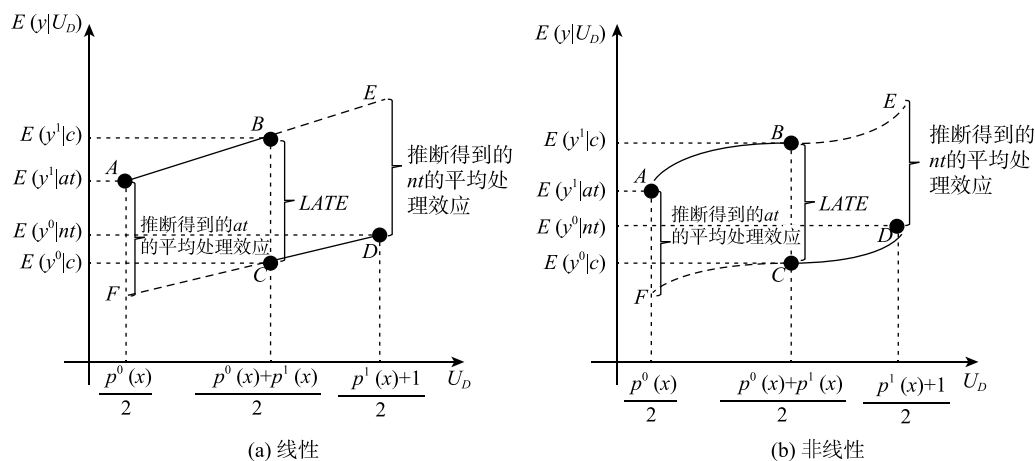
图3 LATE 的外推
