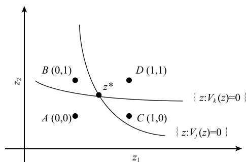
图2 多个工具变量情况下的单调性假设
